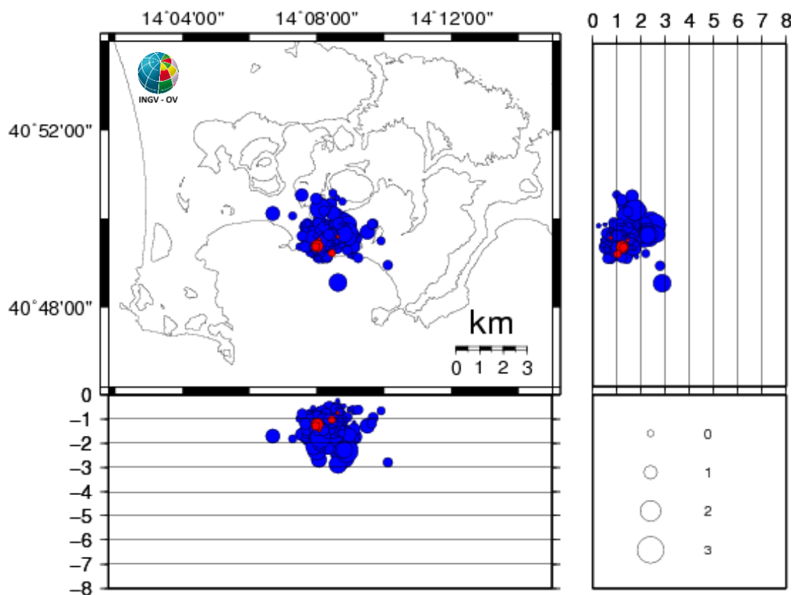
Figura 3.1 - Ipocentri dei terremoti localizzati ai Campi Flegrei negli ultimi 12 mesi (in totale 293). In rosso gli eventi localizzati nell'ultima settimana (in totale 5).
