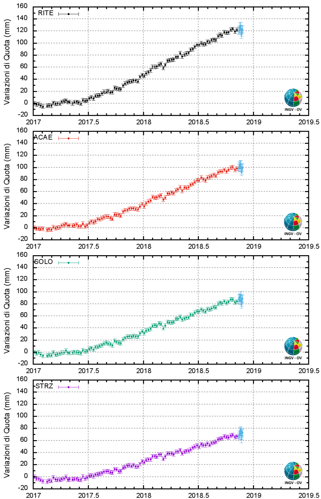
Figura 4.2 - Serie temporali delle variazioni in quota delle stazioni di RITE (Pozzuoli – Rione Terra), ACAE (Accademia Aeronautica), SOLO (Solfatarà) e STRZ (Pozzuoli - Cimitero) dal 01 gennaio 2017 al 25 novembre 2018.
