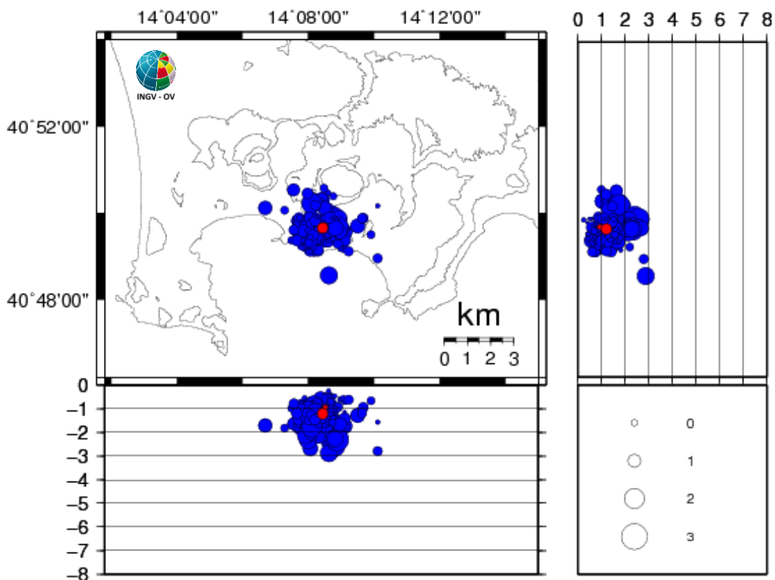
Figura 3.1 - Ipocentri dei terremoti localizzati ai Campi Flegrei negli ultimi 12 mesi (in totale 304). In rosso gli eventi localizzati nell'ultima settimana (in totale 2).
