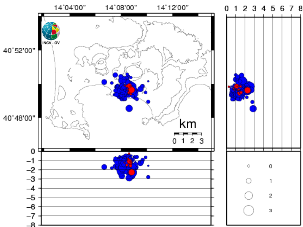
Figura 3.1 - Ipocentri dei terremoti localizzati ai Campi Flegrei negli ultimi 12 mesi (in totale 300). In rosso gli eventi localizzati nell'ultima settimana (in totale 17).
