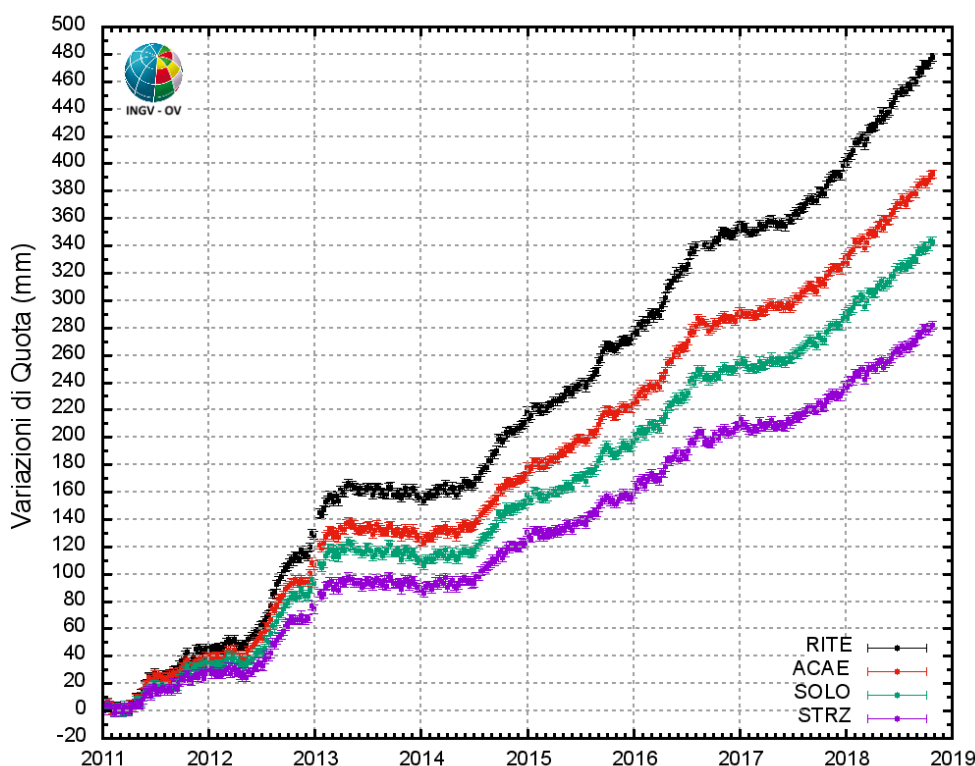
Figura 4.1 - Serie temporali delle variazioni in quota delle stazioni di RITE (Pozzuoli – Rione Terra), ACAE (Accademia Aeronautica), SOLO (Solfatarata) e STRZ (Pozzuoli - Cimitero) dal 01 gennaio 2011 al 27 ottobre 2018.
