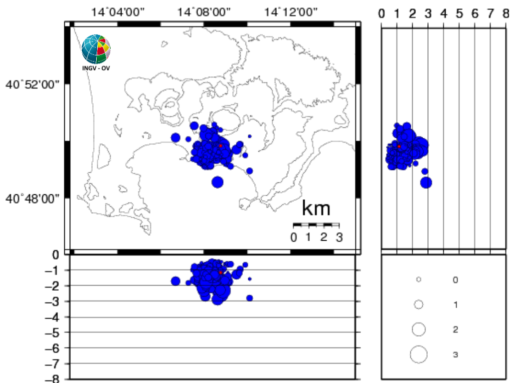
Figura 3.1 - Ipocentri dei terremoti localizzati ai Campi Flegrei negli ultimi 12 mesi (in totale 283). In rosso gli eventi localizzati nell'ultima settimana (in totale 1).
