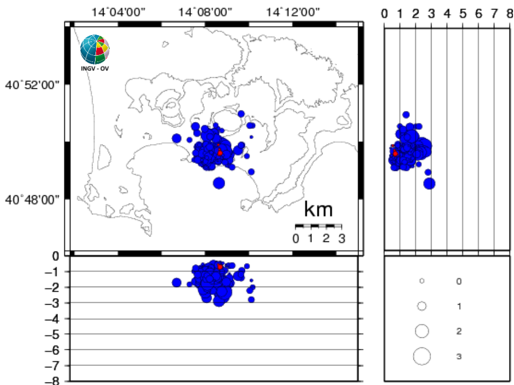
Figura 3.1 - Ipocentri dei terremoti localizzati ai Campi Flegrei negli ultimi 12 mesi (in totale 301). In rosso gli eventi localizzati nell'ultima settimana (in totale 7).
