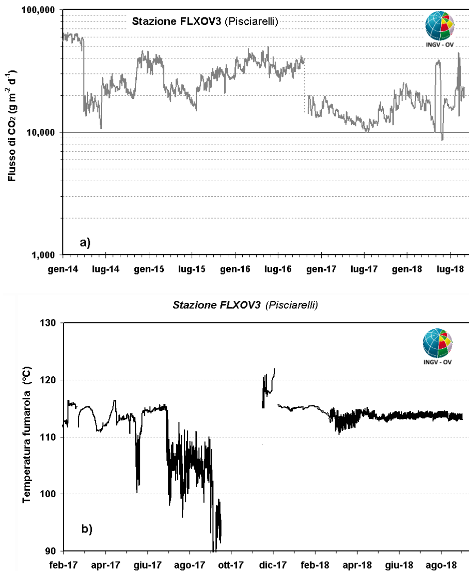
Figura 3.1 - (a) Valori del flusso di CO 2 dal suolo (medie giornaliere) dal 01 gennaio 2014; (b) dettaglio della temperatura della fumarola dal mese di febbraio 2017.
