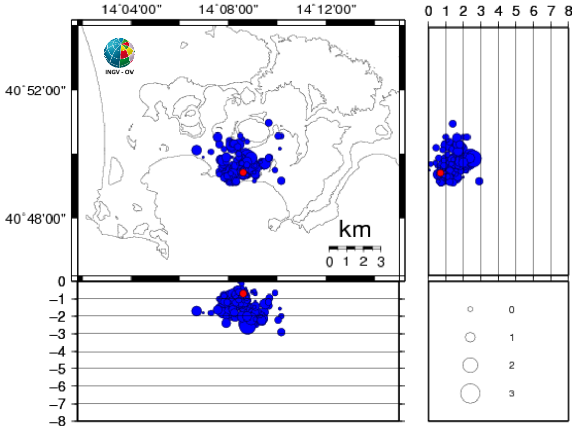
Figura 1.1 - Ipocentri dei terremoti localizzati ai Campi Flegrei negli ultimi 12 mesi (in totale 263). In rosso gli eventi localizzati nell'ultima settimana (in totale 1).
