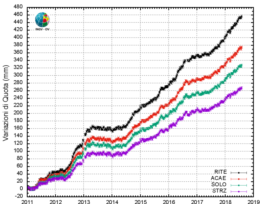
Figura 2.1 - Serie temporali delle variazioni in quota delle stazioni di RITE (Pozzuoli – Rione Terra), ACAE (Accademia Aeronautica), SOLO (Solfatarara) e STRZ (Pozzuoli - Cimitero) dal 01 gennaio 2011 al 04 agosto 2018.
