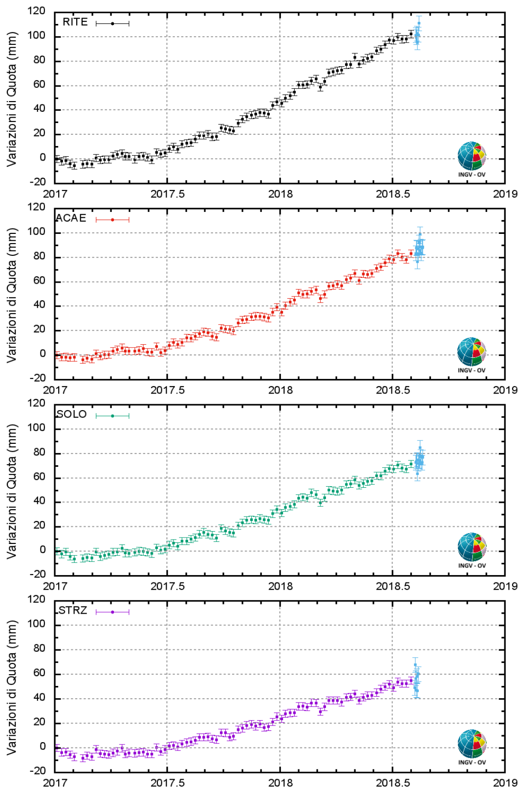
Figura 2.2 - Serie temporali delle variazioni in quota delle stazioni di RITE (Pozzuoli – Rione Terra), ACAE (Accademia Aeronautica), SOLO (Solfatara) e STRZ (Pozzuoli - Cimitero) dal 01 gennaio 2017 al 20 agosto 2018.
