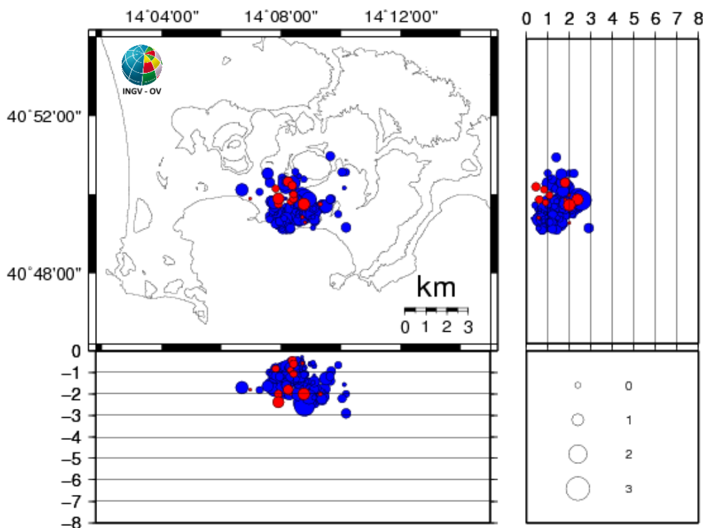
Figura 1.1 - Ipocentri dei terremoti localizzati ai Campi Flegrei negli ultimi 12 mesi (in totale 262). In rosso gli eventi localizzati nell'ultima settimana (in totale 14).
