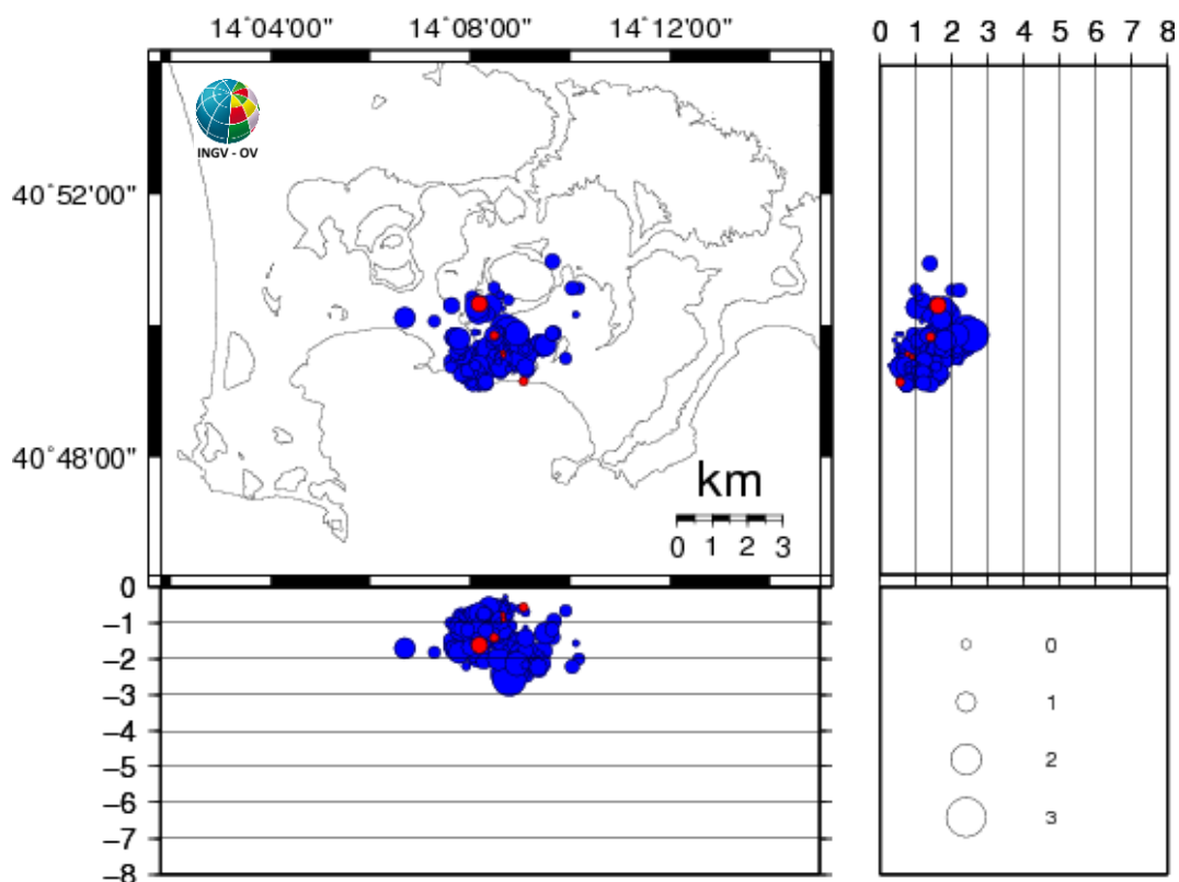
Figura 1.1 - Ipocentri dei terremoti localizzati ai Campi Flegrei negli ultimi 12 mesi (in totale 250). In rosso gli eventi localizzati nell'ultima settimana (in totale 5).
