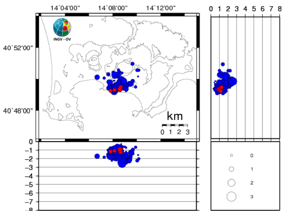
Figura 1.1 - Ipocentri dei terremoti localizzati ai Campi Flegrei negli ultimi 12 mesi (in totale 235). In rosso gli eventi localizzati nell'ultima settimana (in totale 6).
