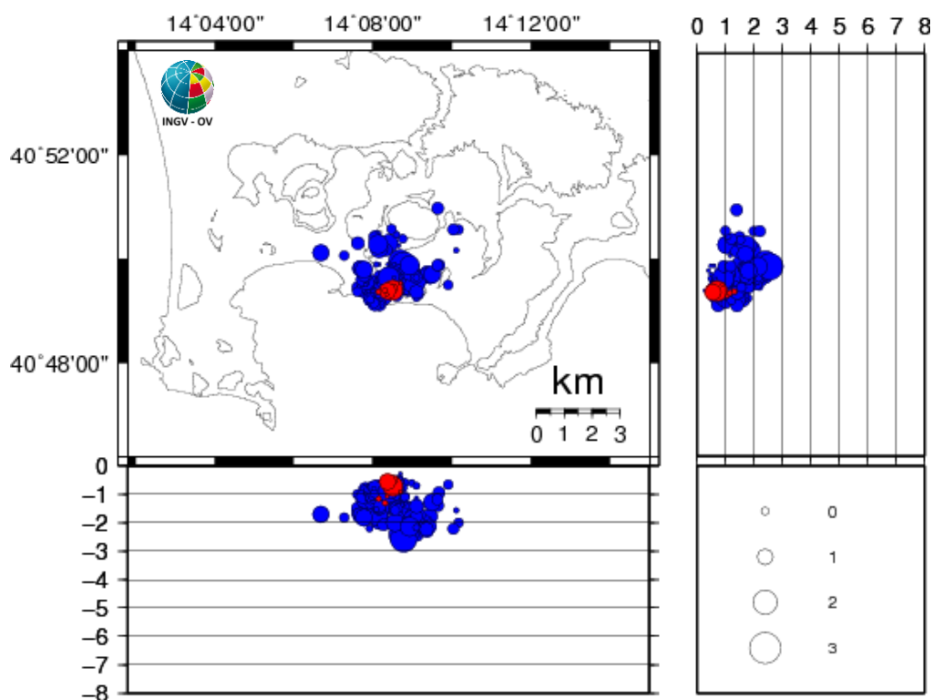
Figura 1.1 - Ipocentri dei terremoti localizzati ai Campi Flegrei negli ultimi 12 mesi (in totale 227). In rosso gli eventi localizzati nell'ultima settimana (in totale 8).
