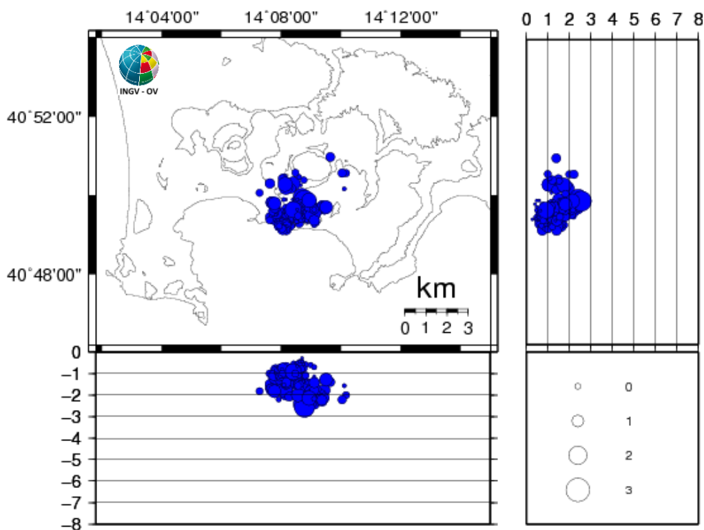
Figura 1.1 - Ipocentri dei terremoti localizzati ai Campi Flegrei negli ultimi 12 mesi (in totale 219).
