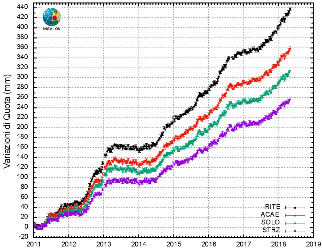
Figura 2.1 - Serie temporali delle variazioni in quota delle stazioni di RITE (Pozzuoli – Rione Terra), ACAE (Accademia Aeronautica), SOLO (Solfatarata) e STRZ (Pozzuoli - Cimitero) dal 01 gennaio 2011 al 05 maggio 2018.
