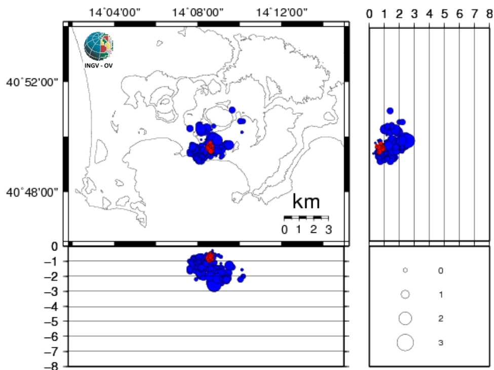
Figura 1.1 - Ipocentri dei terremoti localizzati ai Campi Flegrei negli ultimi 12 mesi (in totale 206). In rosso gli eventi localizzati nell'ultima settimana (in totale 12).
