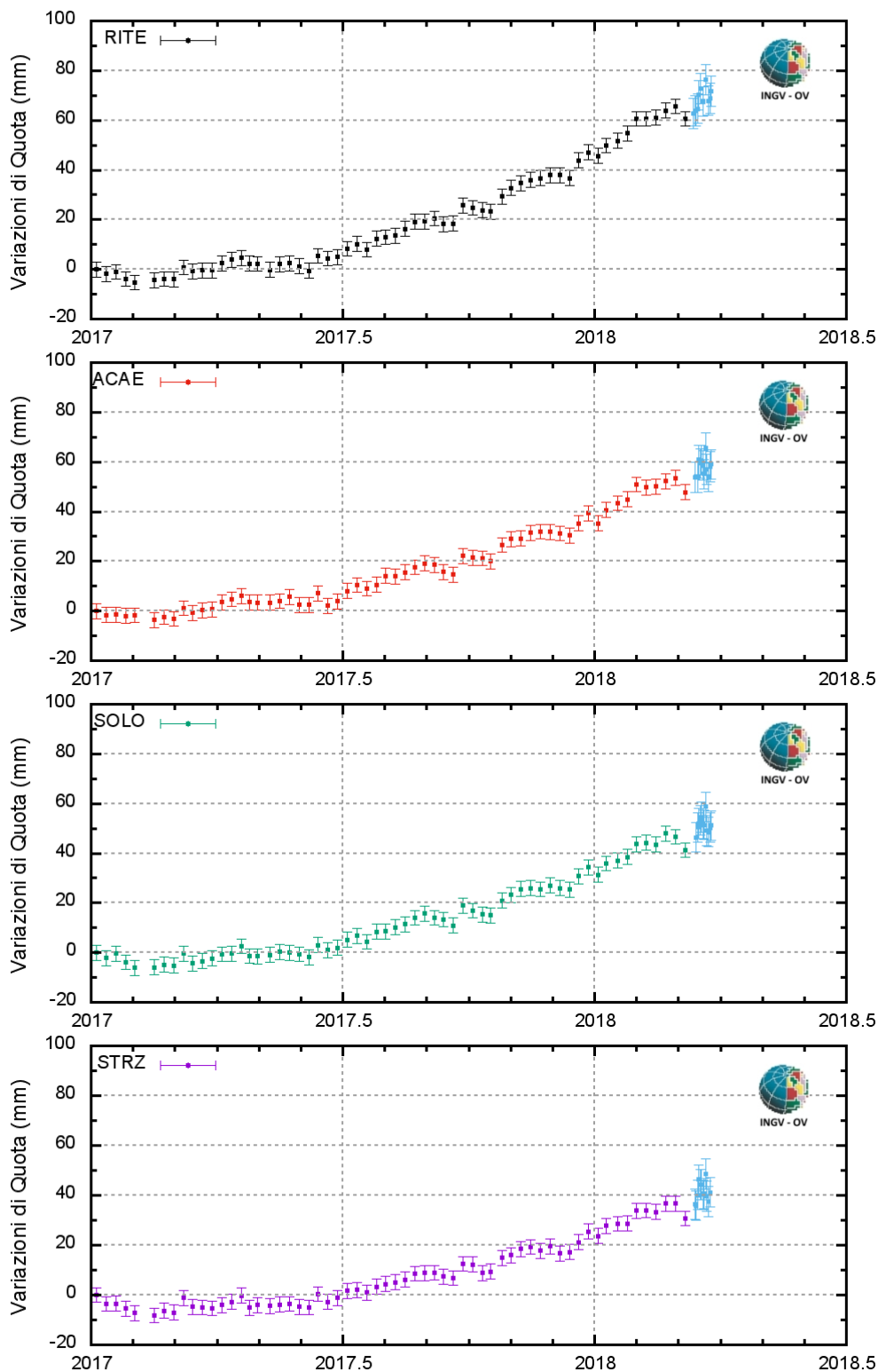
Figura 2.2 - Serie temporali delle variazioni in quota delle stazioni di RITE (Pozzuoli – Rione Terra), ACAE (Accademia Aeronautica), SOLO (Solfatarata) e STRZ (Pozzuoli - Cimitero) dal 01 gennaio 2017 al 26 marzo 2018.
