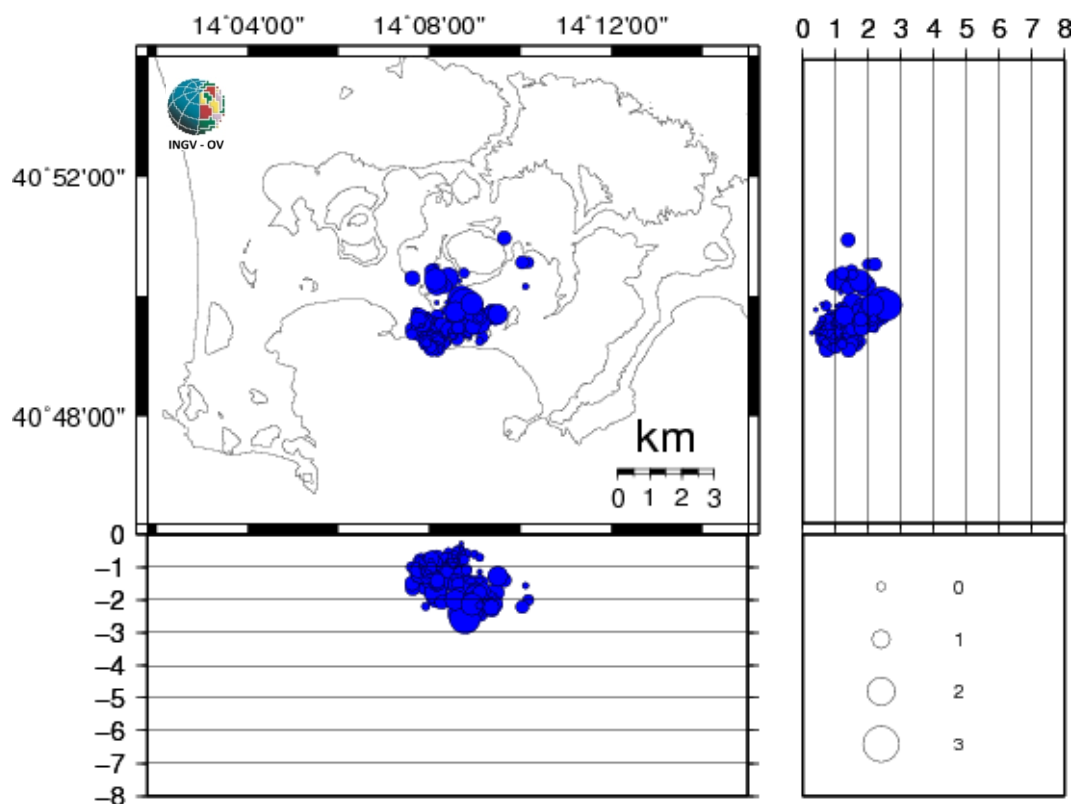
Figura 1.1 - Ipocentri dei terremoti localizzati ai Campi Flegrei negli ultimi 12 mesi (in totale 194).
