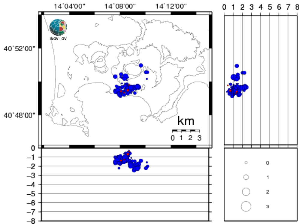
Figura 1.1 - Ipocentri dei terremoti localizzati ai Campi Flegrei negli ultimi 12 mesi (in totale 105). In rosso gli eventi localizzati nell'ultima settimana (in totale 4).
