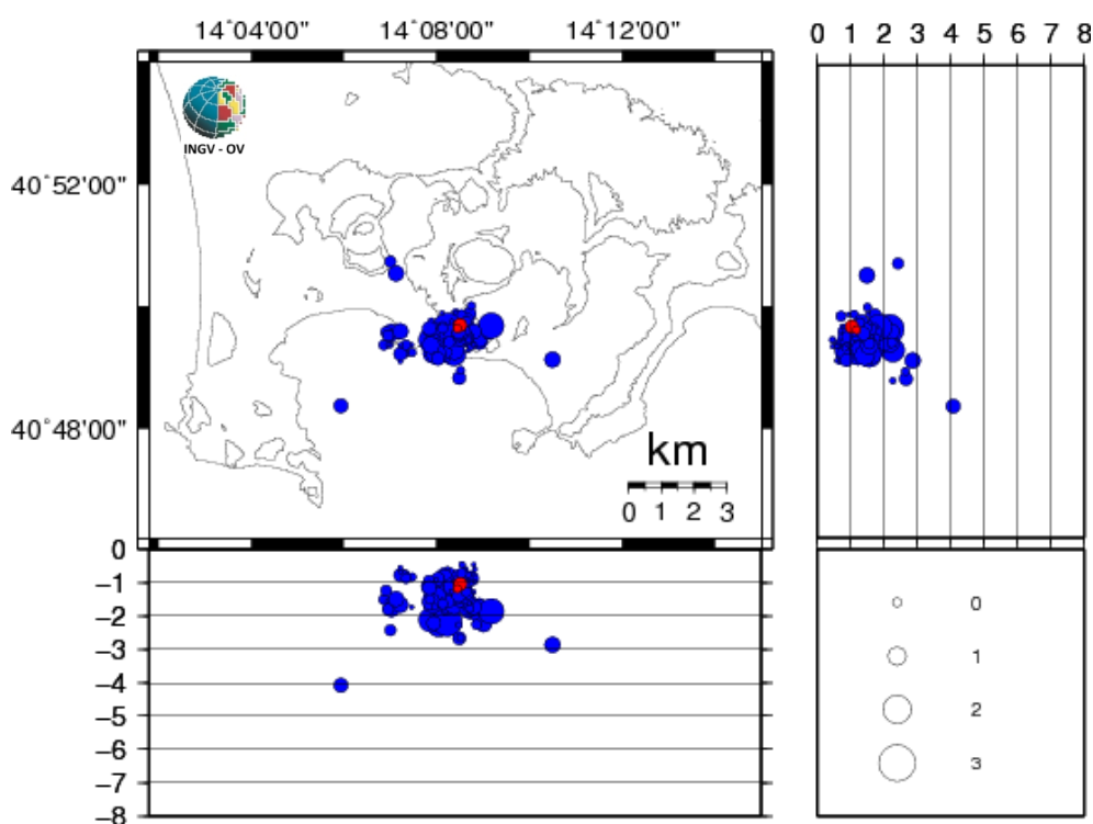
Figura 1.1 - Ipocentri dei terremoti localizzati ai Campi Flegrei negli ultimi 12 mesi (in totale 129). In rosso gli eventi localizzati nell'ultima settimana (in totale 2).
