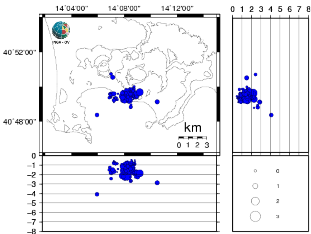
Figura 1.1 - Ipocentri dei terremoti localizzati ai Campi Flegrei negli ultimi 12 mesi (in totale 141).
