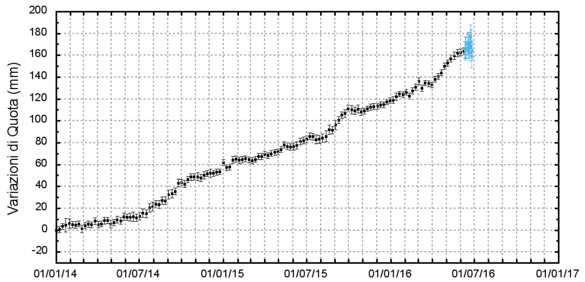
Figura 2 - Serie temporale delle variazioni in quota della stazione di RITE (Pozzuoli) dal 1 gennaio 2011 all'11 giugno 2016 (in alto) e dal 1 gennaio 2014 al 26 giugno 2016 (in basso).
