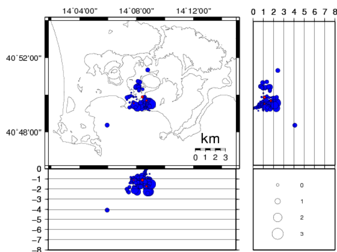
Figura 1 - Ipocentri dei terremoti localizzati ai Campi Flegrei negli ultimi 12 mesi (in totale 125). In rosso gli eventi localizzati nell'ultima settimana.
