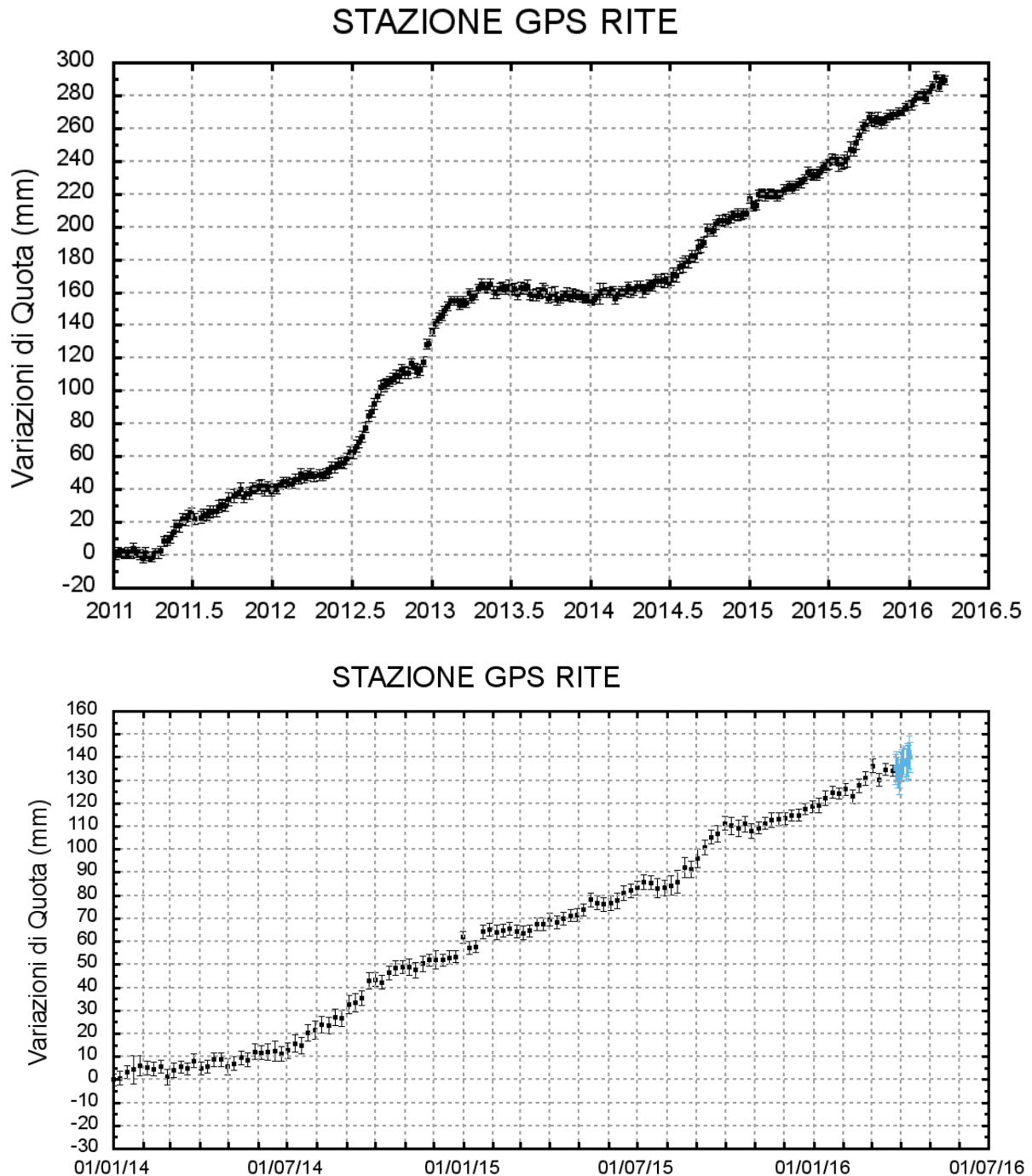
Figura 2 - Serie temporale delle variazioni in quota della stazione di RITE (Pozzuoli) dal 01 gennaio 2011 al 26 marzo 2016 (in alto) e dal 01 gennaio 2014 al 11 aprile 2016 (in basso).
