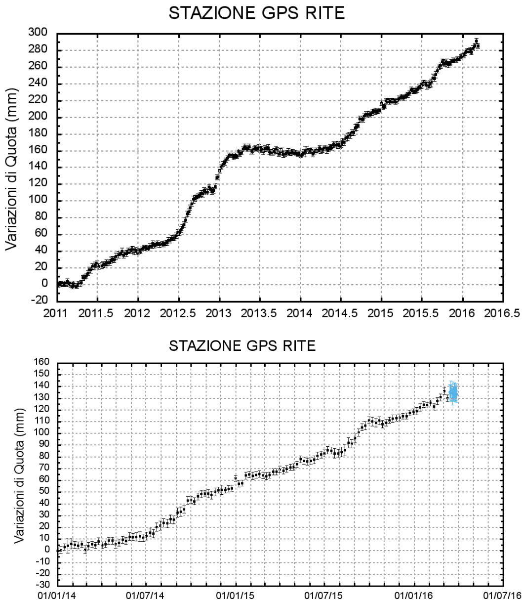
Figura 2 - Serie temporale delle variazioni in quota della stazione di RITE (Pozzuoli) dal 01 gennaio 2011 al 12 marzo 2016 (in alto) e dal 01 gennaio 2014 al 28 marzo 2016 (in basso).
