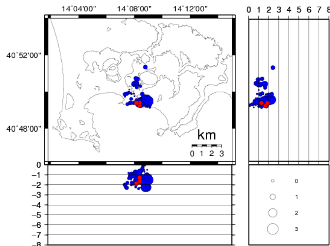
Figura 1 - Ipocentri dei terremoti localizzati ai Campi Flegrei negli ultimi 12 mesi (in totale 116). In rosso gli eventi localizzati nell'ultima settimana.
