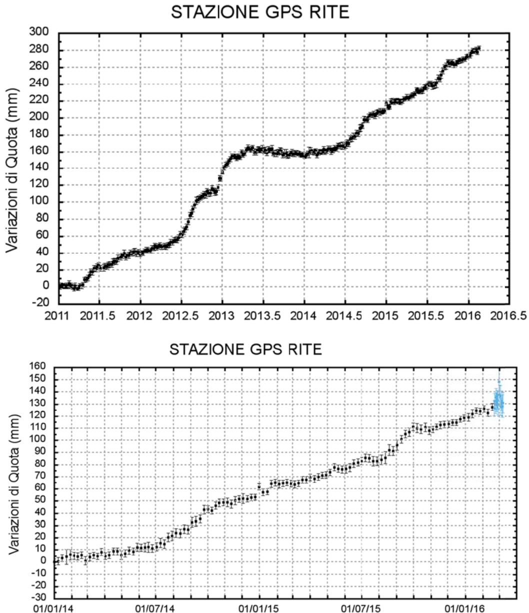
Figura 2 - Serie temporale delle variazioni in quota della stazione di RITE (Pozzuoli) dal 01 gennaio 2011 al 23 gennaio 2016 (in alto) e dal 01 gennaio 2014 al 7 marzo 2016 (in basso).
