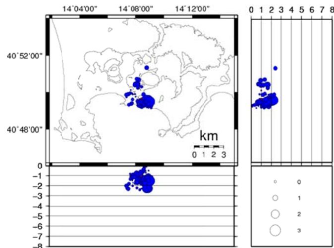
Figura 1 - Ipocentri dei terremoti localizzati ai Campi Flegrei negli ultimi 12 mesi (in totale 110). In rosso gli eventi localizzati nell'ultima settimana.
