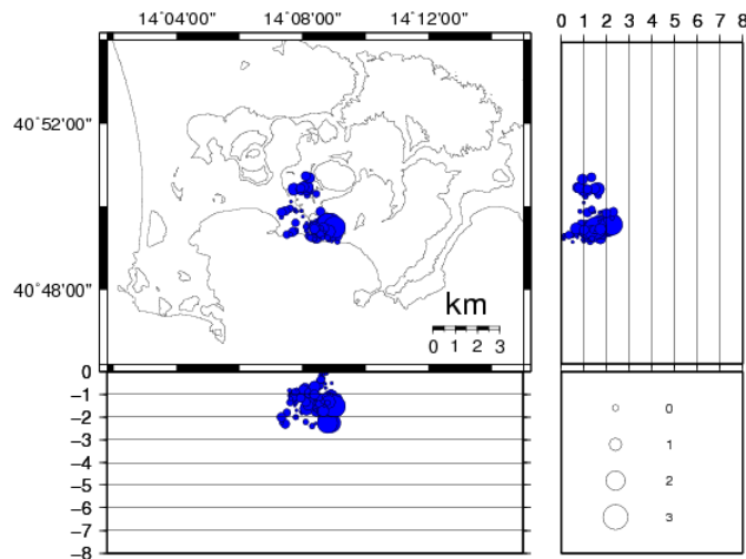
Figura 1 - Ipocentri dei terremoti localizzati ai Campi Flegrei negli ultimi 12 mesi (in totale 104).
