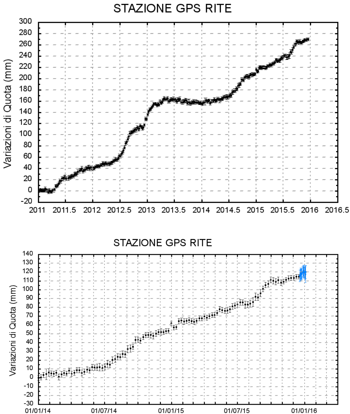
Figura 2 - Serie temporale delle variazioni in quota della stazione di RITE (Pozzuoli) dal 01 gennaio 2011 al 19 dicembre 2015 (in alto) e dal 01 gennaio 2014 al 04 gennaio 2016 (in basso).
