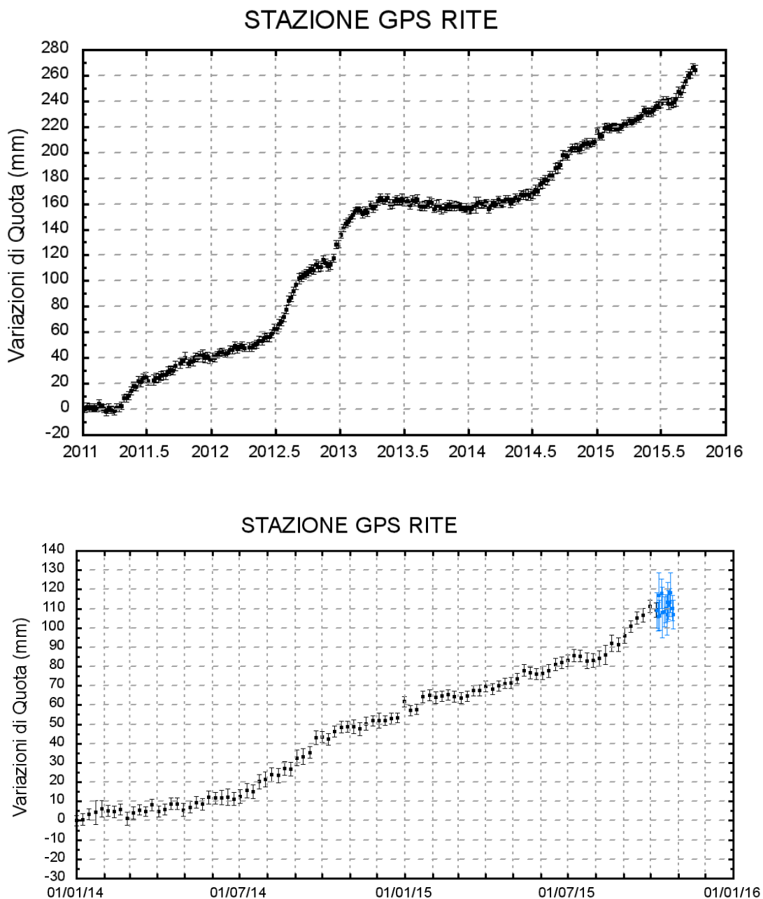
Figura 2 - Serie temporale delle variazioni in quota della stazione di RITE (Pozzuoli) dal 01 gennaio 2011 al 10 ottobre 2015 (in alto) e dal 01 gennaio 2014 al 26 ottobre 2015 (in basso).
