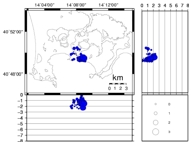
Figura 1 - Ipocentri dei terremoti localizzati ai Campi Flegrei negli ultimi 12 mesi (in totale 99).
