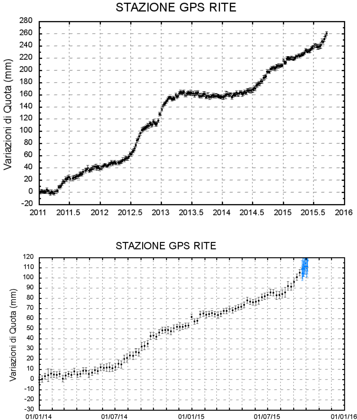
Figura 2 - Serie temporale delle variazioni in quota della stazione di RITE (Pozzuoli) dal 01 gennaio 2011 al 19 settembre 2015 (in alto) e dal 01 gennaio 2014 al 05 ottobre 2015 (in basso).
