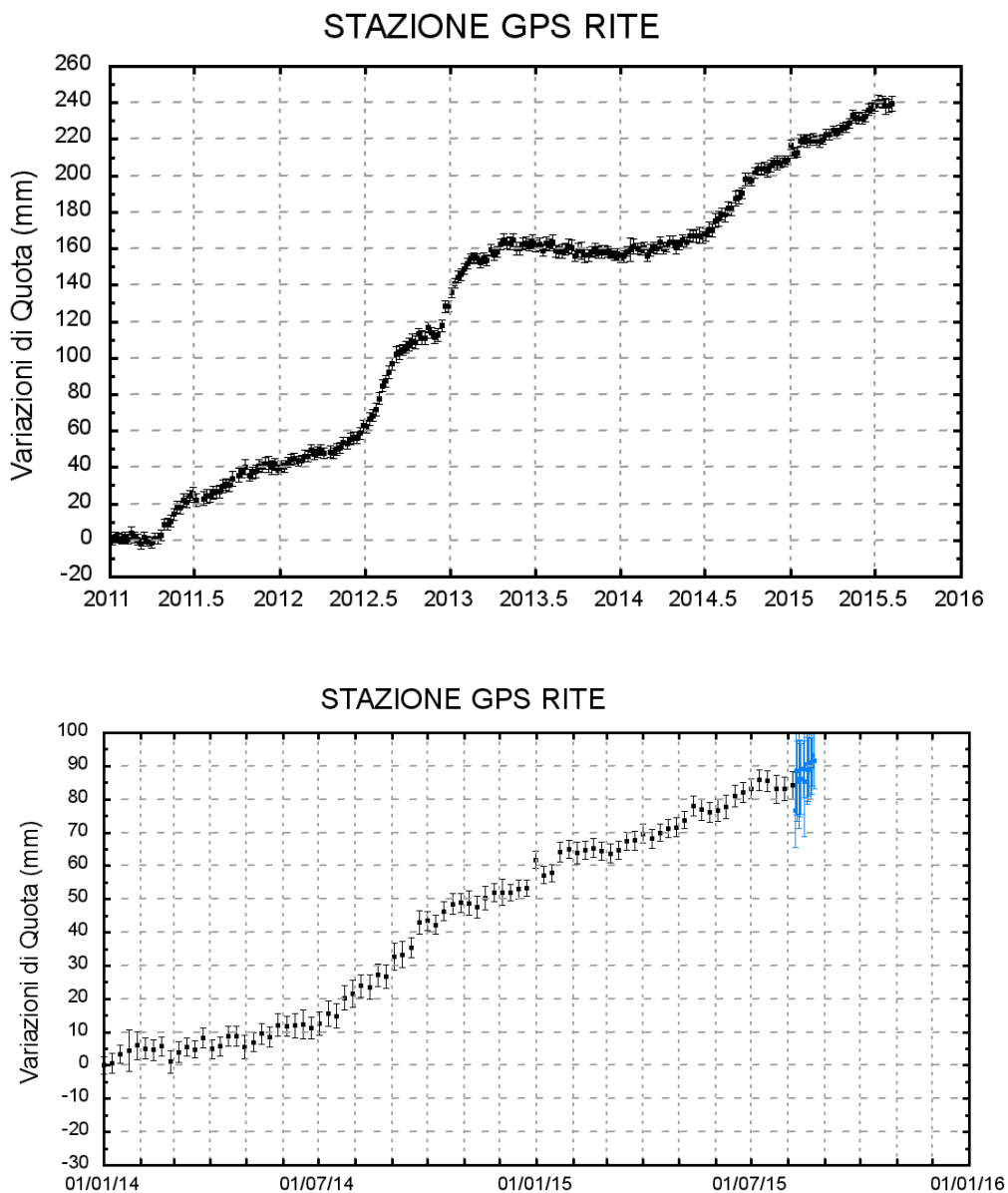
Figura 2 - Serie temporale delle variazioni in quota della stazione di RITE (Pozzuoli) dal 01 gennaio 2011 al 08 agosto 2015 (in alto) e dal 01 gennaio 2014 al 24 agosto 2015 (in basso).
