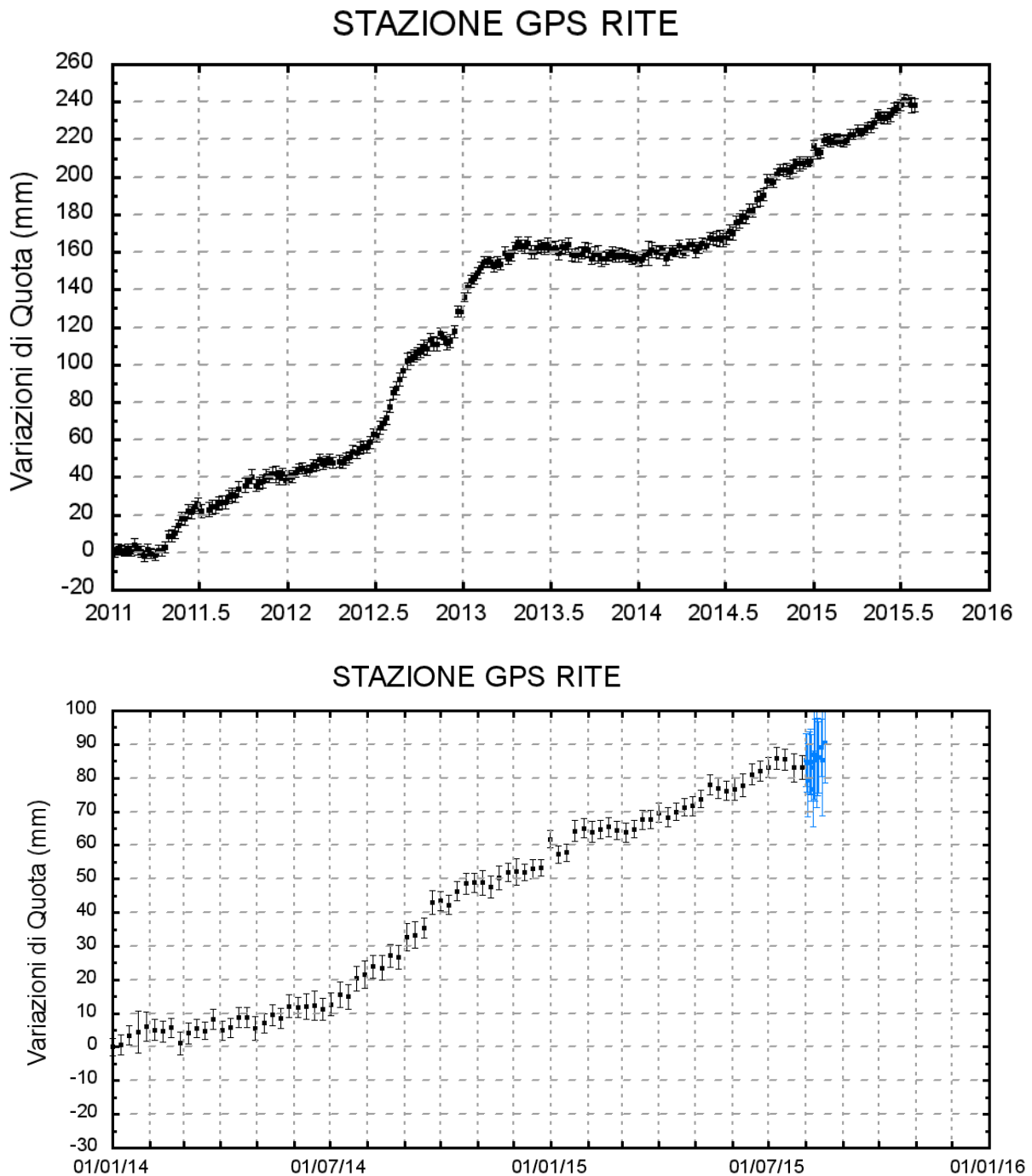
Figura 2 - Serie temporale delle variazioni in quota della stazione di RITE (Pozzuoli) dal 01 gennaio 2011 al 25 luglio 2015 (in alto) e dal 01 gennaio 2014 al 17 agosto 2015 (in basso).
