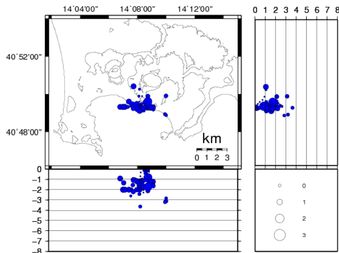
Figura 1 - Ipocentri dei terremoti localizzati ai Campi Flegrei negli ultimi 12 mesi (in totale 107).
