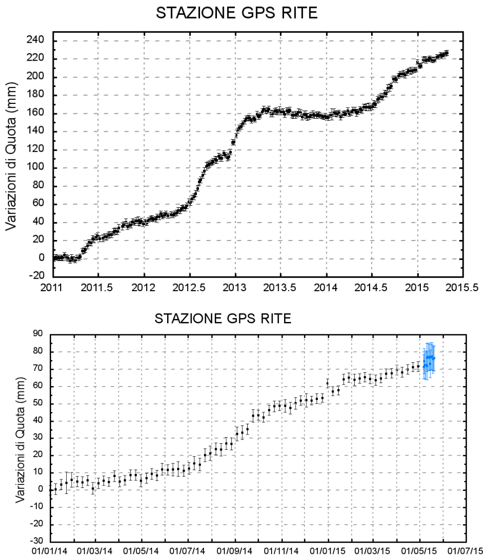
Figura 2 - Serie temporale delle variazioni in quota della stazione di RITE (Pozzuoli) dal 01 gennaio 2011 al 02 maggio 2015 (in alto) e dal 01 gennaio 2014 al 19 maggio 2015 (in basso).
