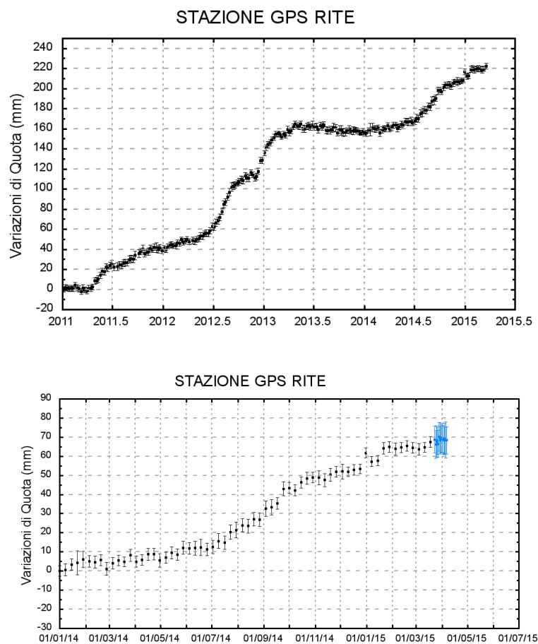
Figura 2 - Serie temporale delle variazioni in quota della stazione di RITE (Pozzuoli) dal 01 gennaio 2011 al 21 marzo 2015 (in alto) e dal 01 gennaio 2014 al 06 aprile 2015 (in basso).
