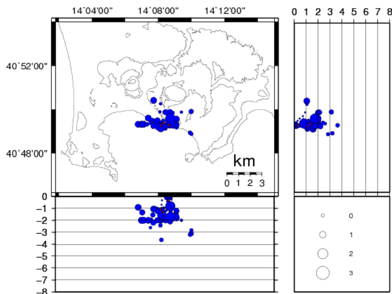
Figura 1 - Ipocentri dei terremoti localizzati ai Campi Flegrei negli ultimi 12 mesi (in totale 102). In rosso gli eventi localizzati nell'ultima settimana.
