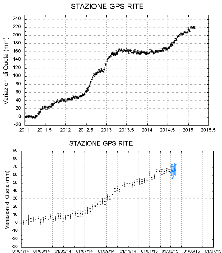
Figura 2 - Serie temporale delle variazioni in quota della stazione di RITE (Pozzuoli) dal 01 gennaio 2011 al 28 febbraio 2015 (in alto) e dal 01 gennaio 2014 al 16 marzo 2015 (in basso).
