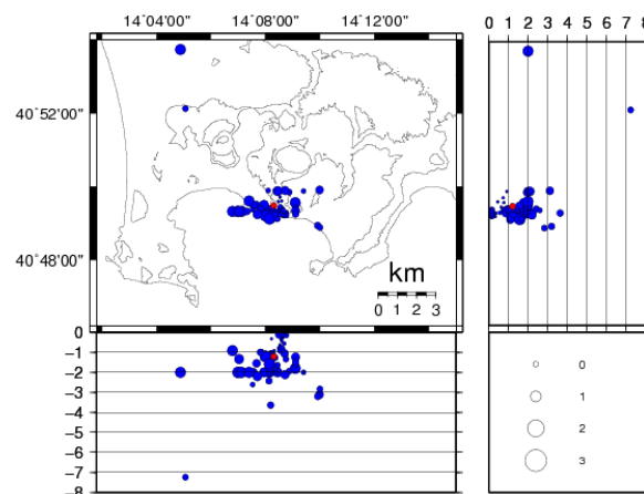
Figura 1 - Ipocentri dei terremoti localizzati ai Campi Flegrei negli ultimi 12 mesi (in totale 72). Quelli avvenuti nell'ultima settimana sono colorati in rosso (in totale 1).
