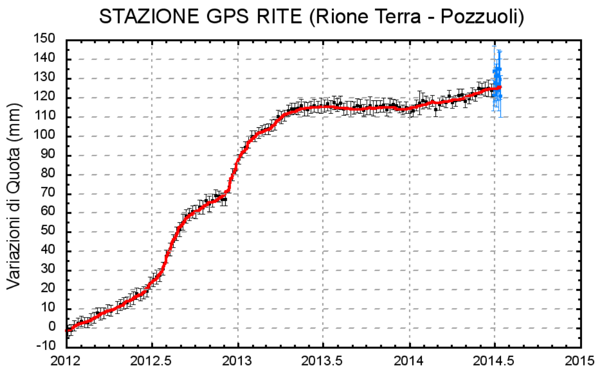
Figura 2 - Serie temporale delle variazioni in quota della stazione di RITE (Pozzuoli) dal 01 gennaio 2012 al 14 luglio 2014.
