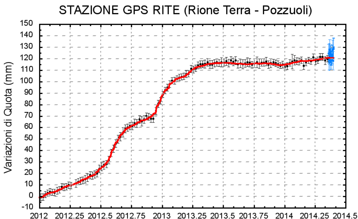
Fig. 2.1: Serie temporale delle variazioni in quota della stazione di RITE (Pozzuoli) dal 01 gennaio 2012 al 26 maggio 2014.
