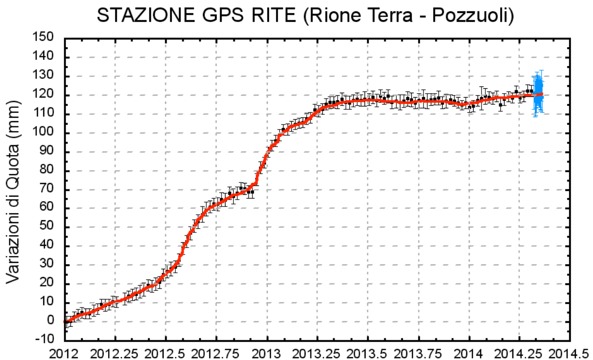
Fig. 2.1: Serie temporale delle variazioni in quota della stazione di RITE (Pozzuoli) dal 01 gennaio 2012 al 12 maggio 2014.
