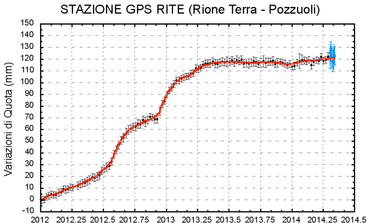
Fig. 2.1: Serie temporale delle variazioni in quota della stazione di RITE (Pozzuoli) dal 01 gennaio 2012 al 05 maggio 2014.
