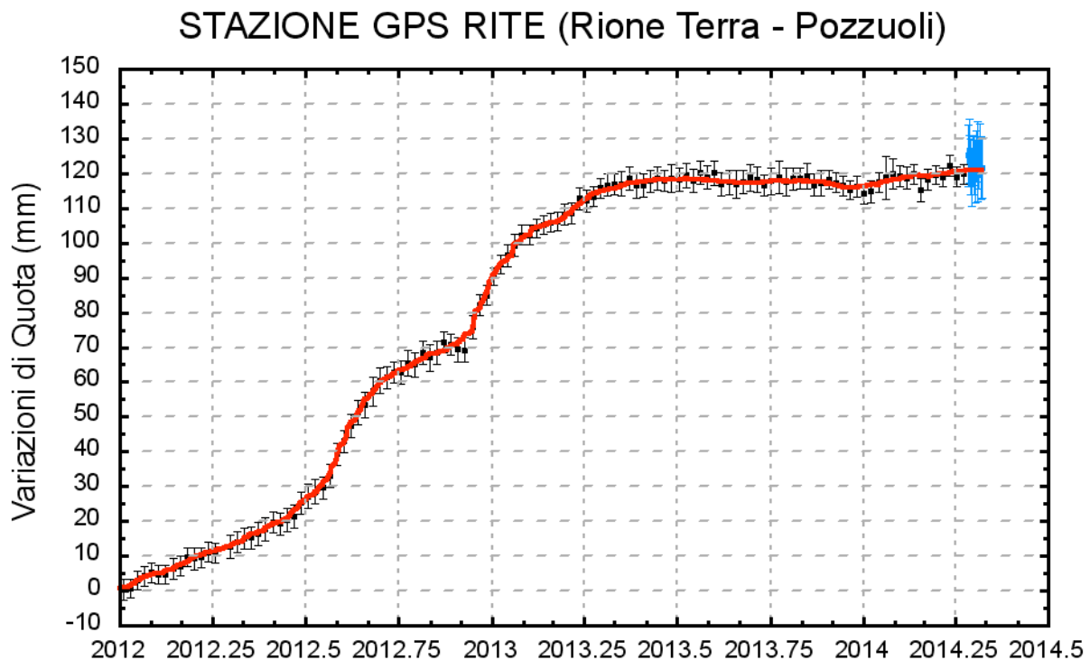
Fig. 2.1: Serie temporale delle variazioni in quota della stazione di RITE (Pozzuoli) dal 01 gennaio 2012 al 28 aprile 2014.
