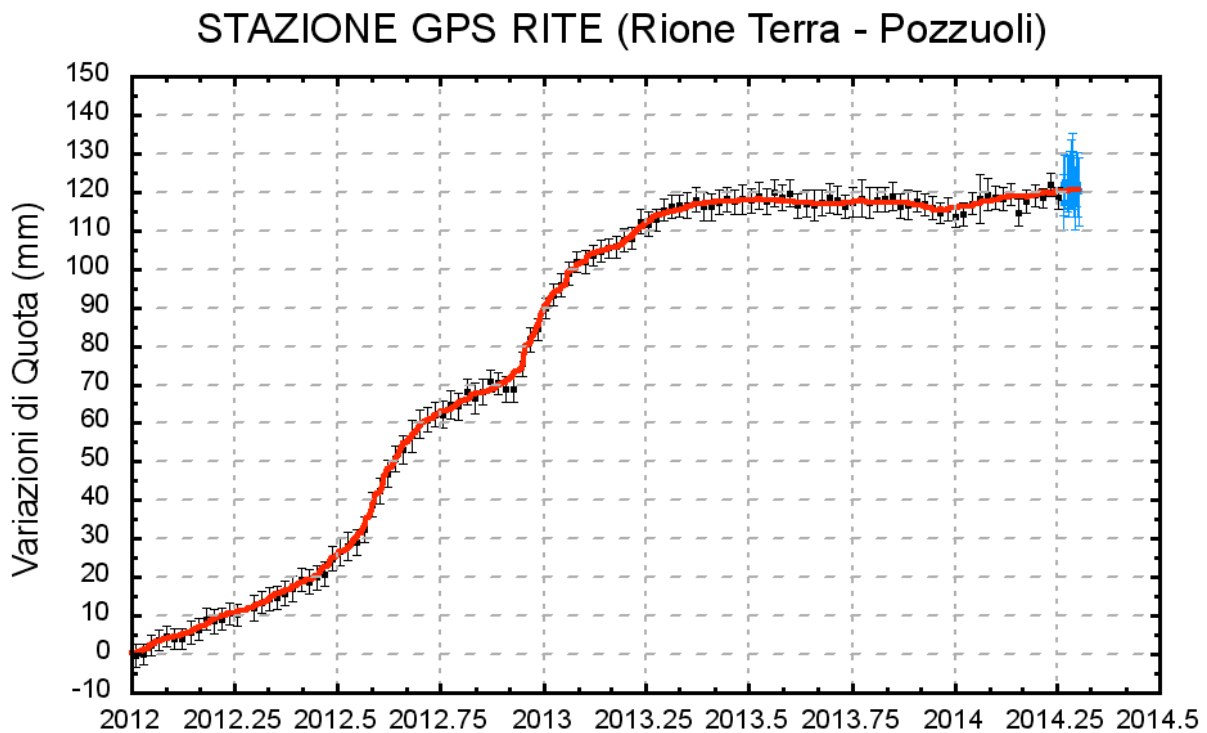
Fig. 2.2.1: Serie temporale delle variazioni in quota della stazione di RITE (Pozzuoli) dal 01 gennaio 2012 al 20 aprile 2014.
