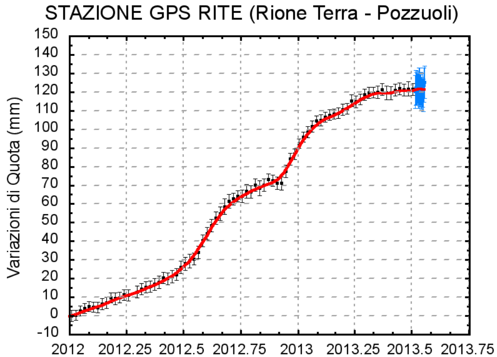
Fig. 2.1: Serie temporale delle variazioni in quota della stazione di RITE (Pozzuoli) dal 01 gennaio 2012 al 22 luglio 2013.
