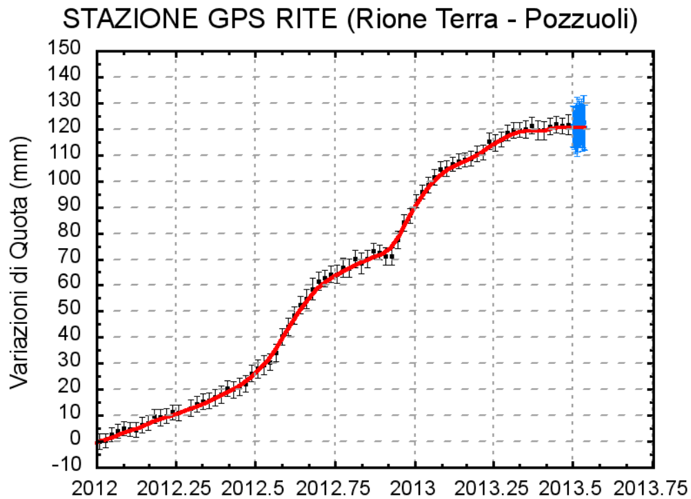
Fig. 2.1: Serie temporale delle variazioni in quota della stazione di RITE (Pozzuoli) dal 01 gennaio 2012 al 15 luglio 2013.
