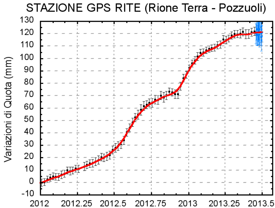
Fig. 2.1: Serie temporale delle variazioni in quota della stazione di RITE (Pozzuoli) dal 01 gennaio 2012 al 01 luglio 2013.
