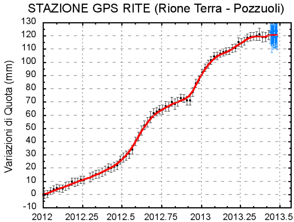
Fig. 2.1: Serie temporale delle variazioni in quota della stazione di RITE (Pozzuoli) dal 01 gennaio 2012 al 25 giugno 2013.
