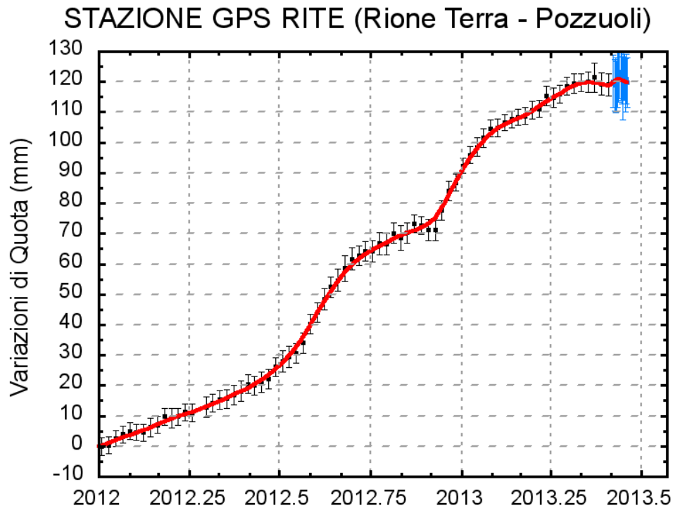
Fig. 2.1: Serie temporale delle variazioni in quota della stazione di RITE (Pozzuoli) dal 01 gennaio 2012 al 17 giugno 2013.
