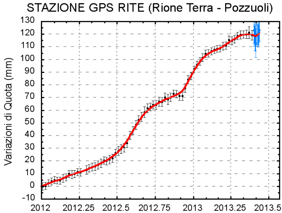
Fig. 2.1: Serie temporale delle variazioni in quota della stazione di RITE (Pozzuoli) dal 01 gennaio 2012 al 09 giugno 2013.
