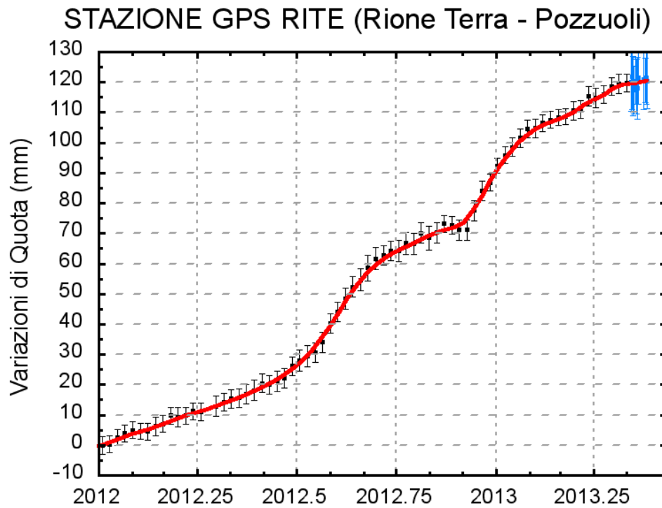
Fig. 2.1: Serie temporale delle variazioni in quota della stazione di RITE (Pozzuoli) dal 01 gennaio 2012 al 20 maggio 2013.
