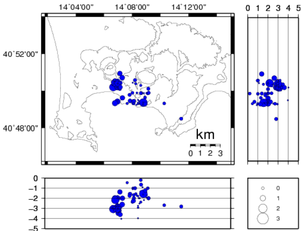
Fig. 1.1 Nella mappa sono rappresentati in colore blu gli ipocentri localizzati negli ultimi 12 mesi (99).
