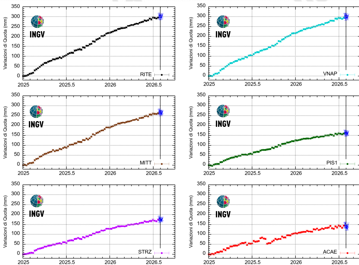
Figura 4.5 - Serie temporali delle variazioni in quota delle stazioni di RITE (Pozzuoli - Rione Terra), VNAP (Pozzuoli - Via Napoli), MITT (Pozzuoli - Porto), PIS1 (Pisciarelli), STRZ (Pozzuoli - Cimitero) e ACAE (Accademia Aeronautica) dal 01/01/2025 al 09/08/2026, con le discontinuità cosismiche corrette (valori preliminari). Elaborazione dati in modalità differenziale singola baseline con software GNSS Spider.
