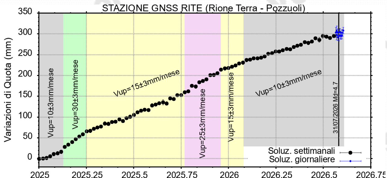
Figura 4.3 – Serie temporale delle variazioni in quota della stazione GNSS di RITE dal 01/01/2025 al 09/08/2026, con la discontinuità cosismica corretta (valori preliminari). Elaborazione dati in modalità differenziale singola baseline con software GNSS Spider.
