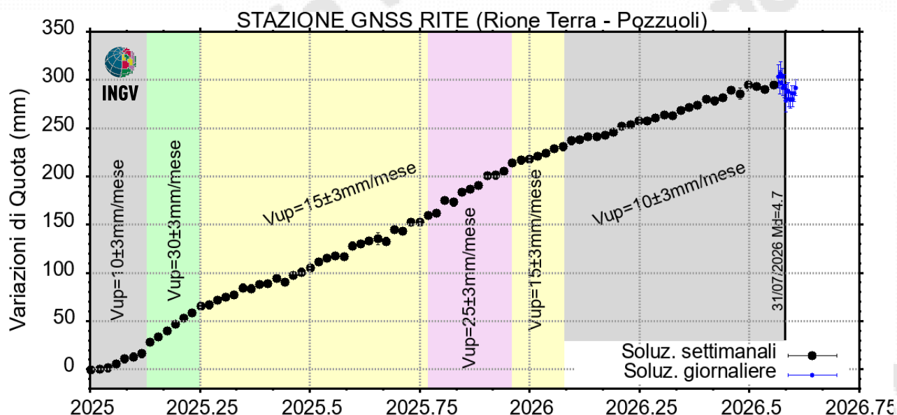
Figura 4.2 – Serie temporale delle variazioni in quota della stazione GNSS di RITE dal 01/01/2025 al 09/08/2026, con la discontinuità cosismica registrata il 31/07. Elaborazione dati in modalità differenziale singola baseline con software GNSS Spider.
