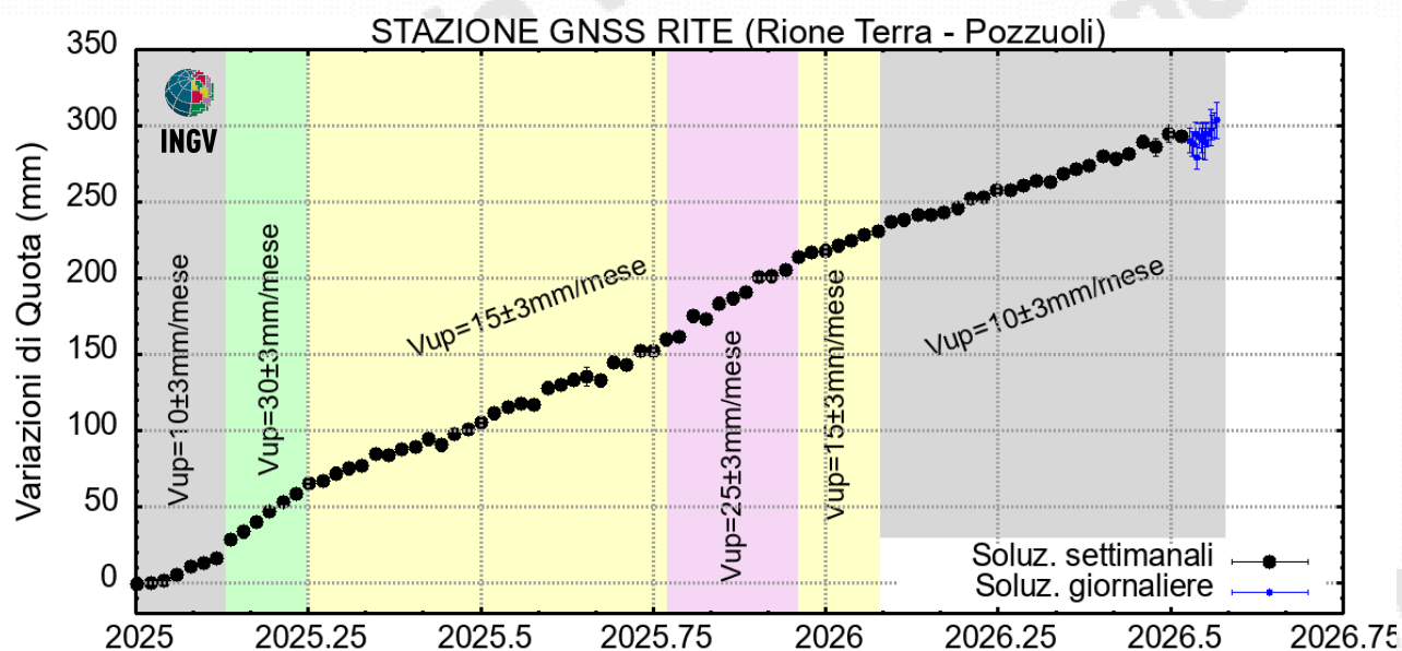
Figura 4.2 – Serie temporale delle variazioni in quota della stazione GNSS di RITE dal 01/01/2025 al 26/07/2026. Elaborazione dati in modalità differenziale singola baseline con software GNSS Spider.
