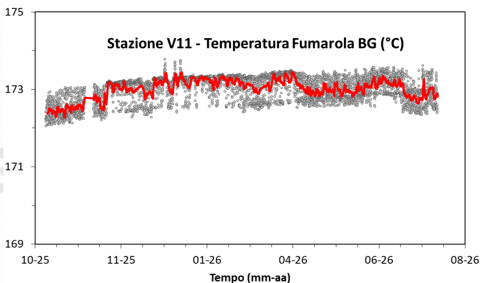
Figura 5.3 Valori della temperatura della fumarola BG misurati dalla stazione V11 installata nel cratere della Solfatara a pochi metri dalla fumarola principale BG.
