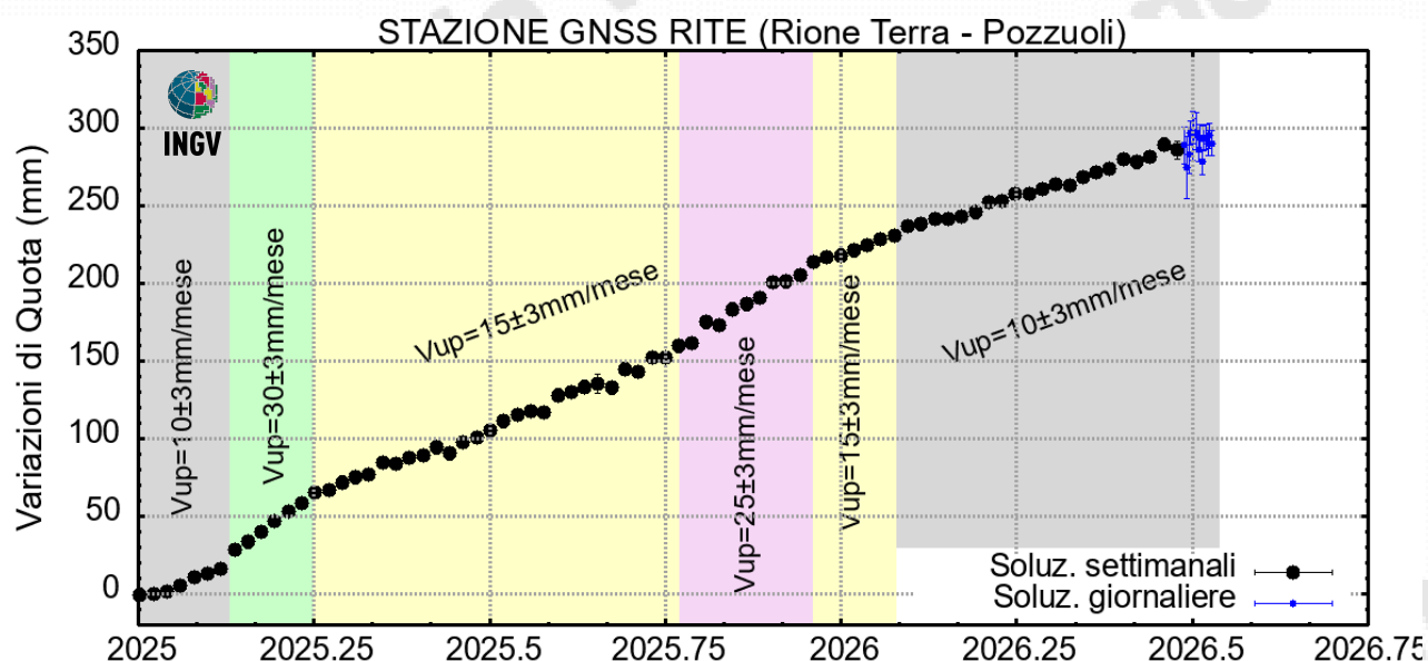
Figura 4.2 – Serie temporale delle variazioni in quota della stazione GNSS di RITE dal 01/01/2025 al 12/07/2026. Elaborazione dati in modalità differenziale singola baseline con software GNSS Spider.
