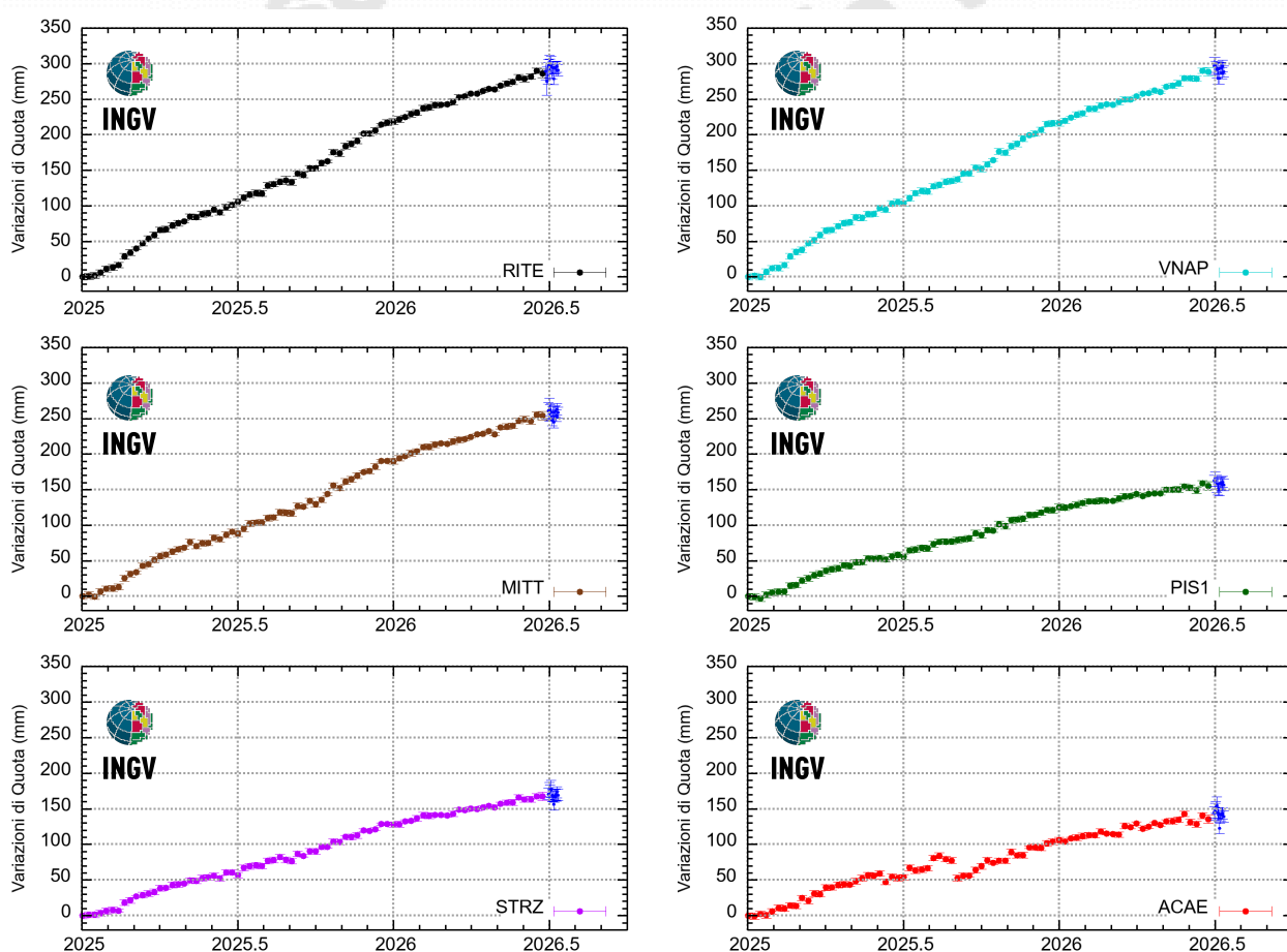
Figura 4.3 - Serie temporali delle variazioni in quota delle stazioni di RITE (Pozzuoli - Rione Terra), VNAP (Pozzuoli - Via Napoli), MITT (Pozzuoli - Porto), PIS1 (Pisciarelli), STRZ (Pozzuoli - Cimitero) e ACAE (Accademia Aeronautica) dal 01/01/2025 al 12/07/2026. Elaborazione dati in modalità differenziale singola baseline con software GNSS Spider.
