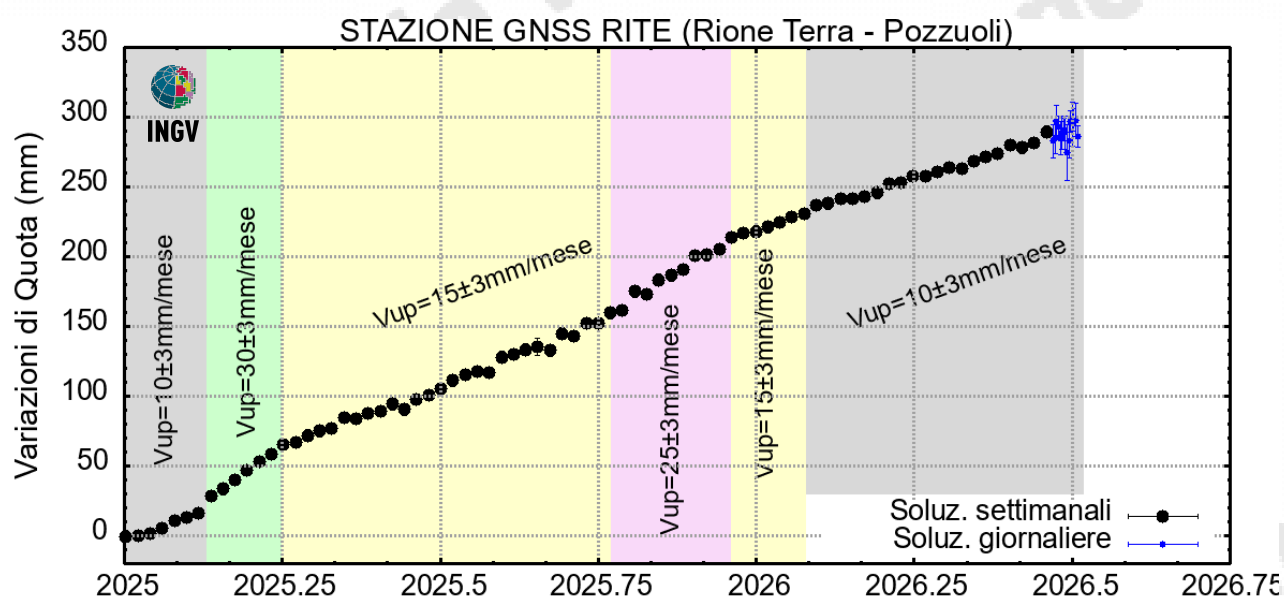
Figura 4.2 – Serie temporale delle variazioni in quota della stazione GNSS di RITE dal 01/01/2025 al 05/07/2026. Elaborazione dati in modalità differenziale singola baseline con software GNSS Spider.
