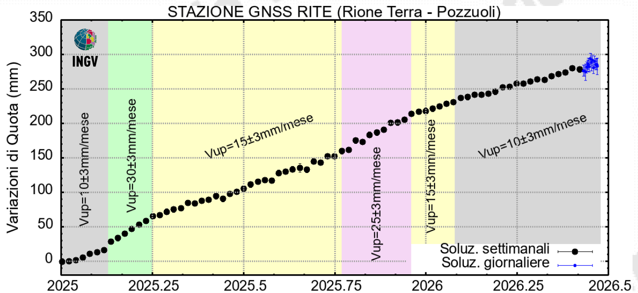
Figura 4.2 – Serie temporale delle variazioni in quota della stazione GNSS di RITE dal 01/01/2025 al 21/06/2026. Elaborazione dati in modalità differenziale singola baseline con software GNSS Spider.
