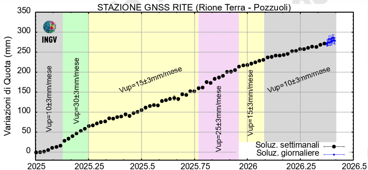
Figura 4.2 – Serie temporale delle variazioni in quota della stazione GNSS di RITE dal 01/01/2025 al 31/05/2026. Elaborazione dati in modalità differenziale singola baseline con software GNSS Spider.
