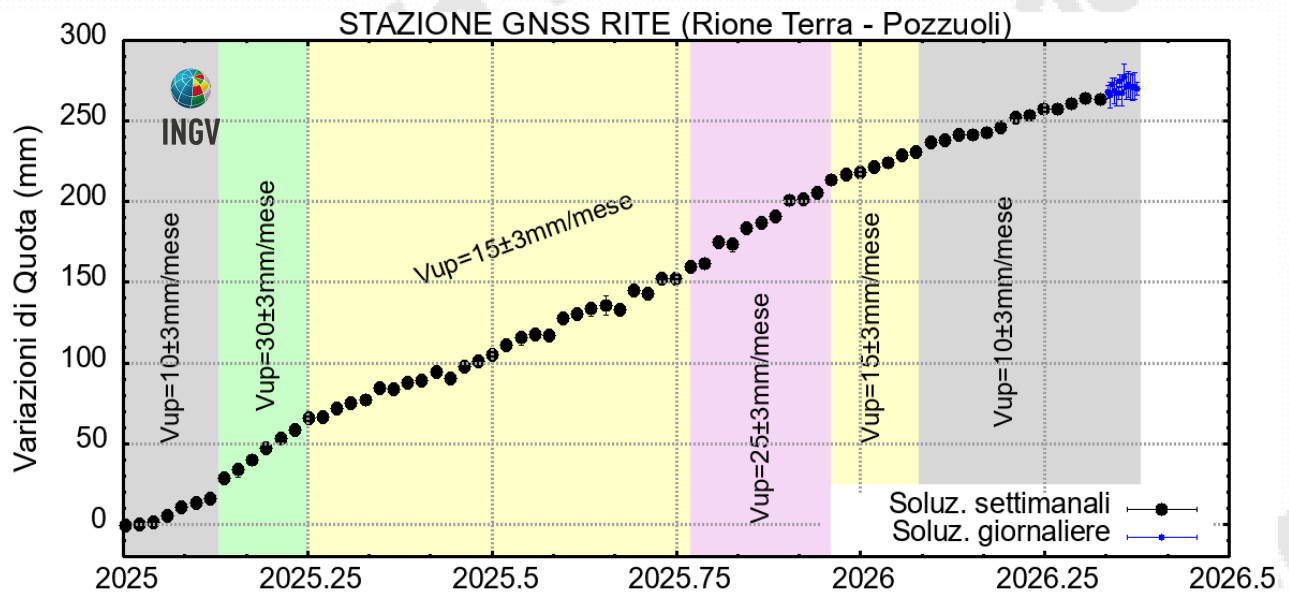
Figura 4.2 – Serie temporale delle variazioni in quota della stazione GNSS di RITE dal 01/01/2025 al 17/05/2026. Elaborazione dati in modalità differenziale singola baseline con software GNSS Spider.
