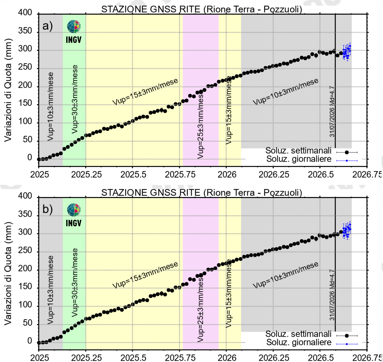
Figura 4.2 – Serie temporale delle variazioni in quota della stazione GNSS di RITE dal 01/01/2025 al 30/08/2026, con (a) e senza (b) la discontinuità cosismica del 31/07. Elaborazione dati in modalità differenziale singola baseline con software GNSS Spider.
